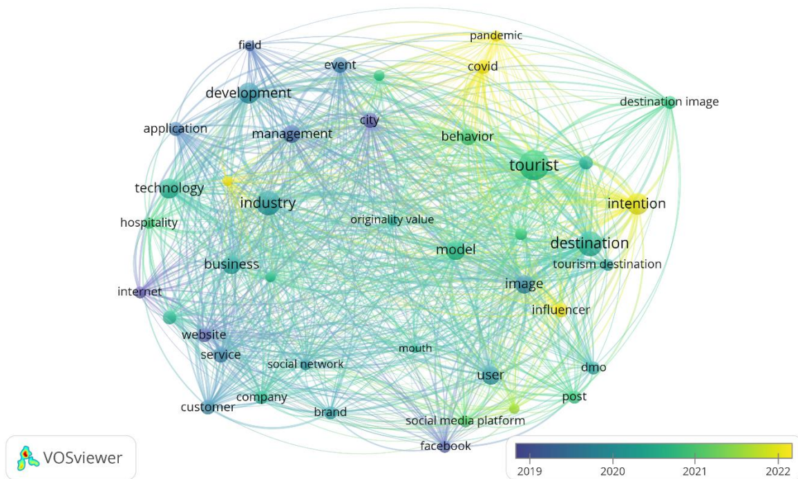
Gambar 2. Visualisasi Overlay
